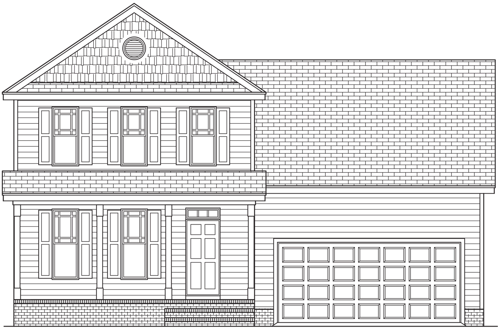
Elevation A
